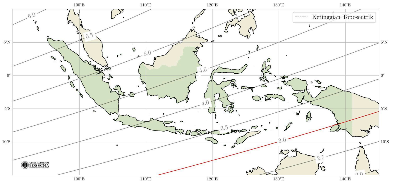
Gambar 4. Peta Ketinggian Bulan saat Matahari terbenam pada Sabtu, 6 Juli 2024
