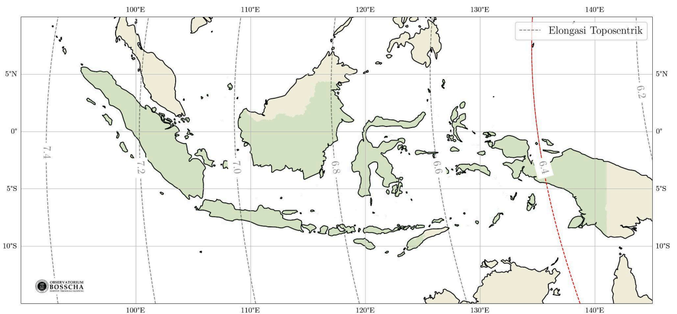
Gambar 3. Peta Elongasi toposentrik Bulan dan Matahari saat Matahari terbenam pada Sabtu, 6 Juli 2024
