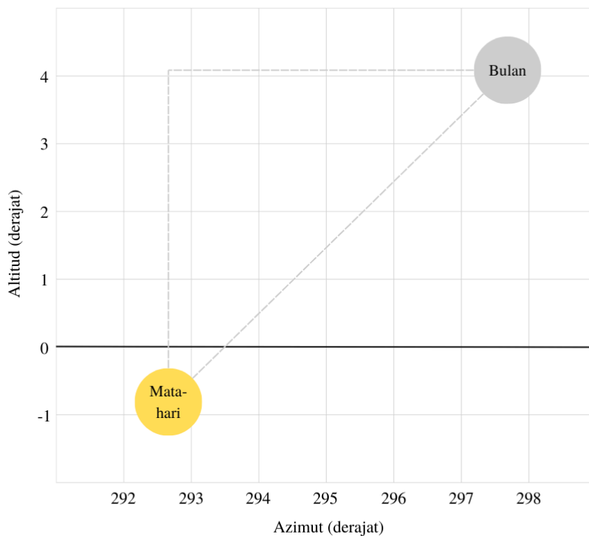
Gambar 1. Konfigurasi Bulan dan Matahari saat Matahari terbenam pada Sabtu, 6 Juli 2024
