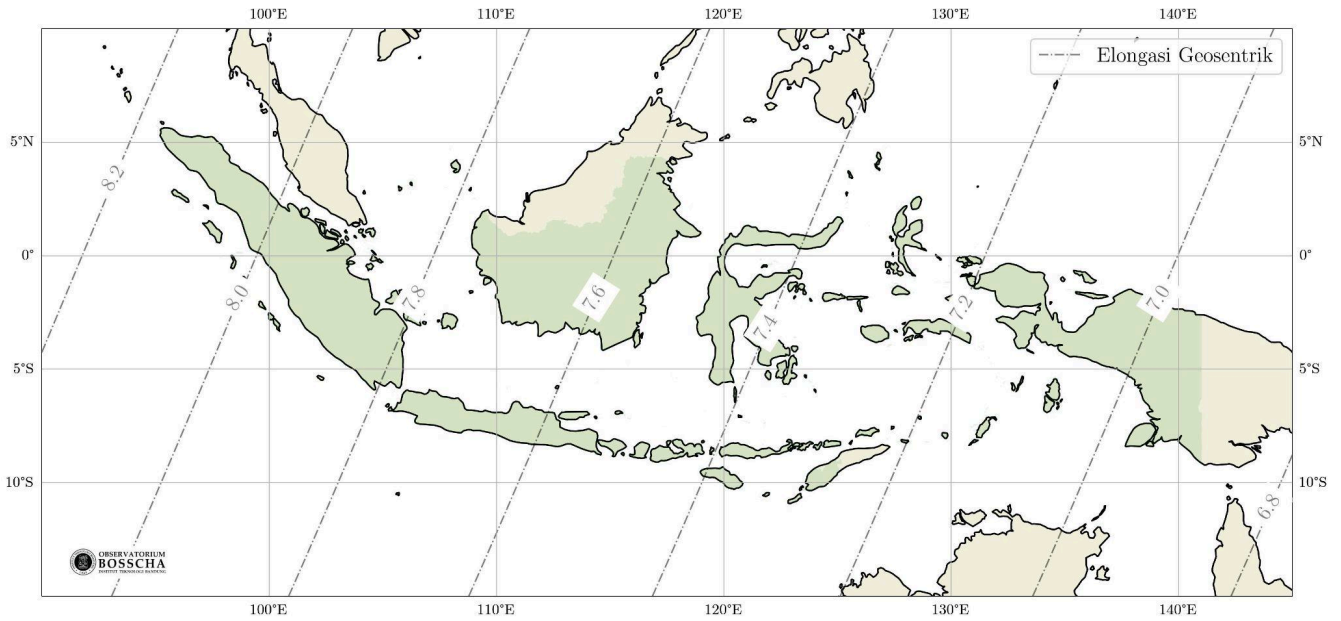
Gambar 2. Peta Elongasi geosentrik Bulan dan Matahari saat Matahari terbenam pada Sabtu, 6 Juli 2024
